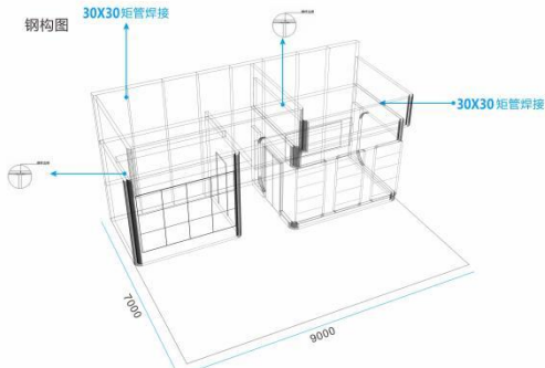
钢构图
